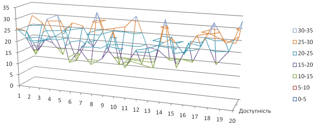
Рисунок 4. Класифікаційна сітка
