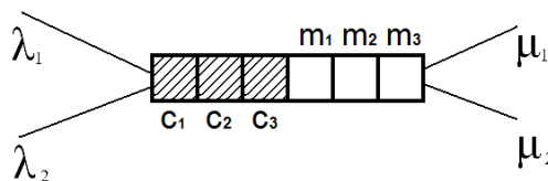
Рисунок 2 – Структура комутатора з трьома каналами передачі і трьома елементами пам'яті.
