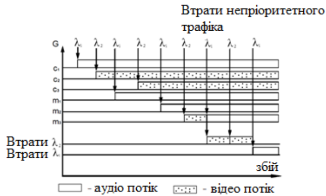
Рисунок 3 – Часова діаграма переходів станів
